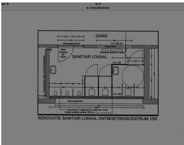
RENOVATIE SANITAIR LOKAAL ONTMOETINGSCENTRUM 1/50 AANGEPAST PLAN - 24.03.2016
