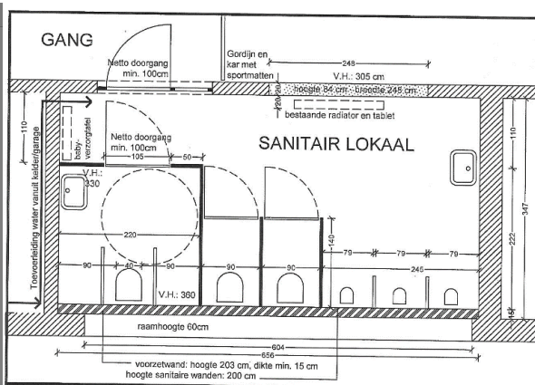
RENOVATIE SANITAIR LOKAAL ONTMOETINGSCENTRUM 1/50 AANGEPAST PLAN - 24.03.2016
